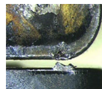
従来品 低抵抗プレーカ
